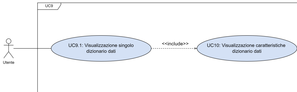
Figura 3.10: UC9 – Sottocasi d'uso
