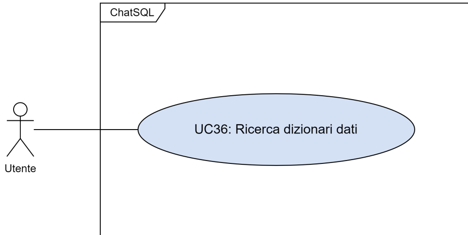
Figura 3.32: UC36
