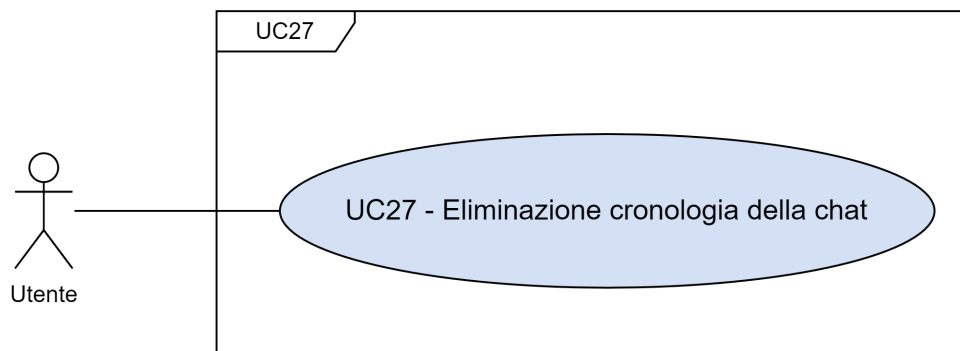
Figura 3.27: UC27
