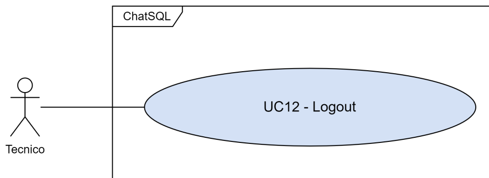
Figura 3.12: UC12
