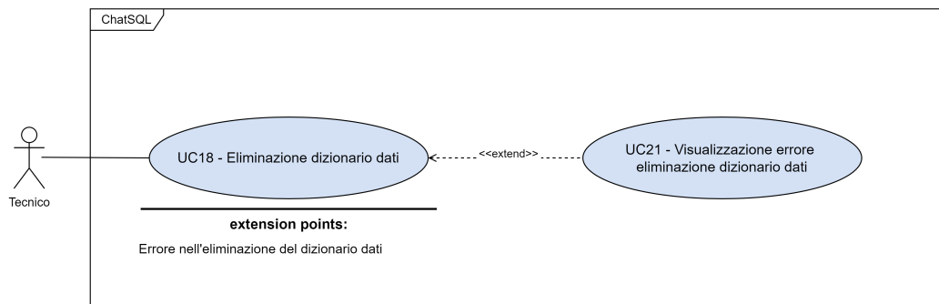
Figura 3.19: UC18
