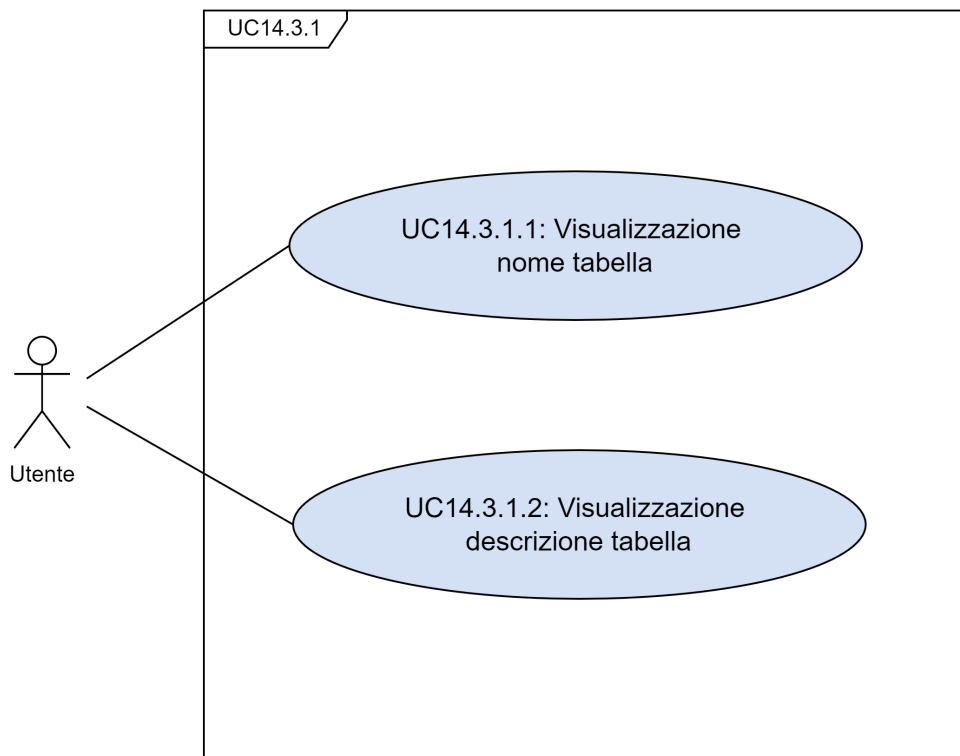
Figura 3.18: UC14.3.1 – Sottocasi d'uso
