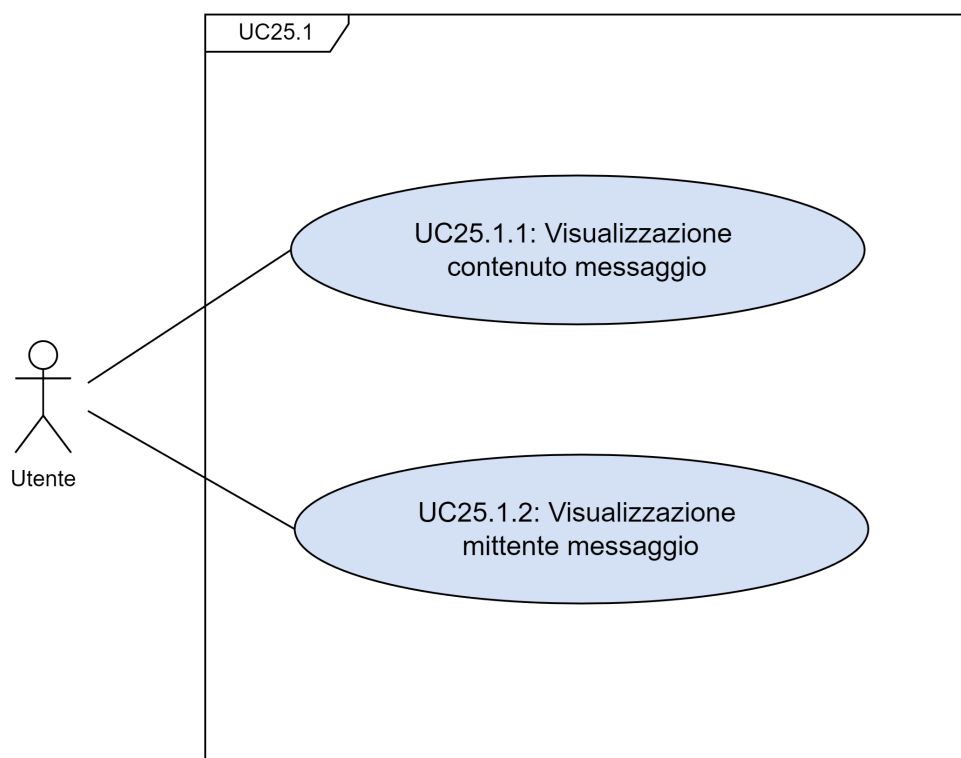
Figura 3.25: UC25.1 – Sottocasi d’uso
