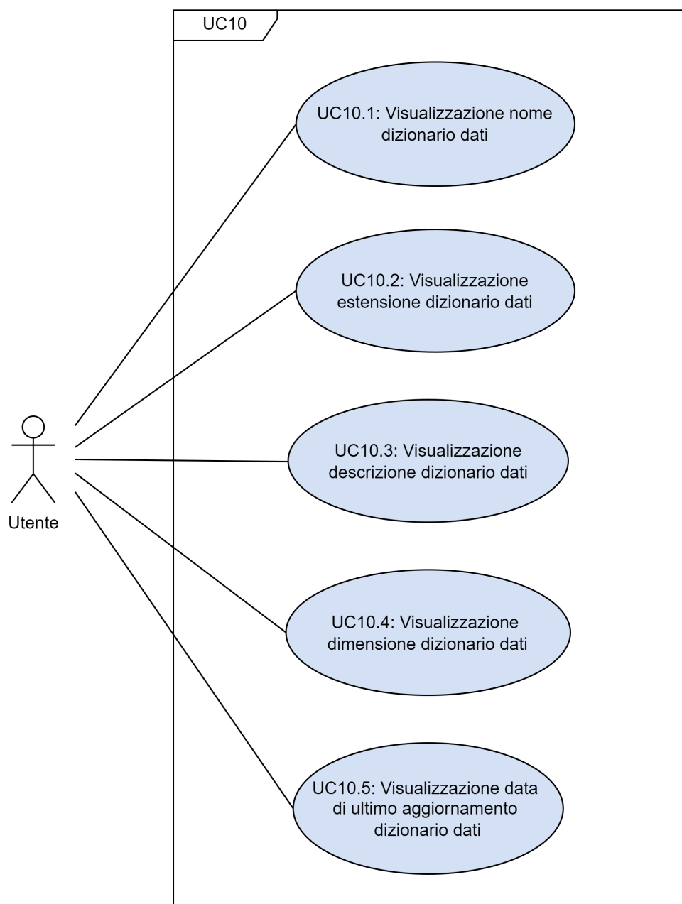
Figura 3.11: UC10 - Sottocasi d'uso
