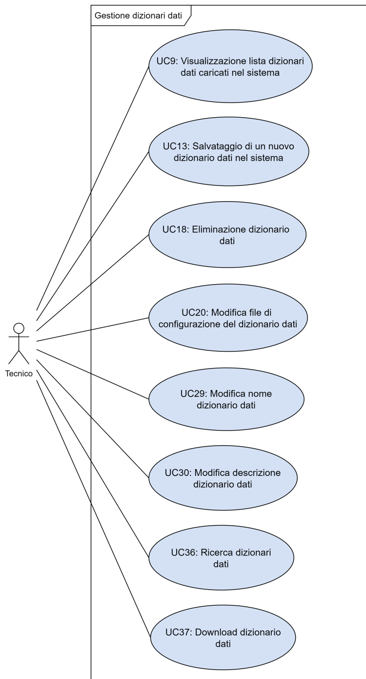
Figura 3.13: Diagramma gestione dizionari
