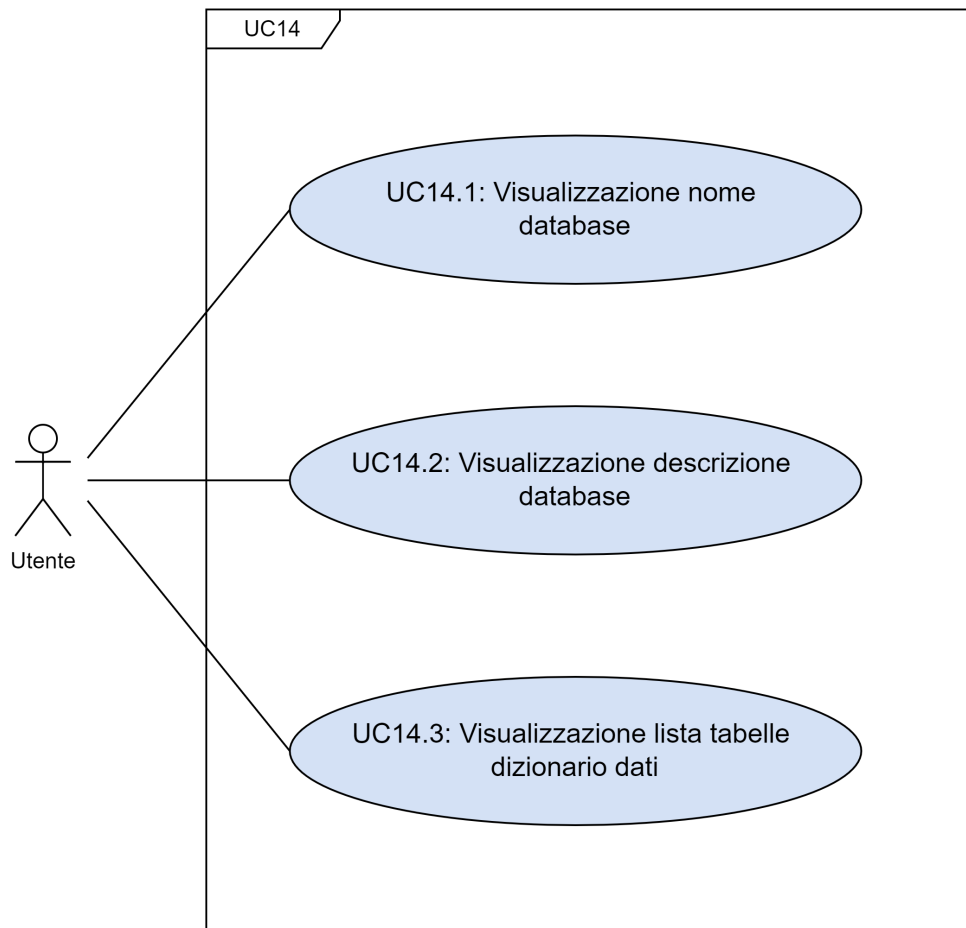
Figura 3.16: UC14 – Sottocasi d'uso
