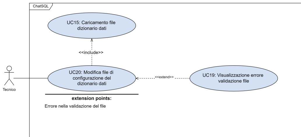
Figura 3.21: UC20
