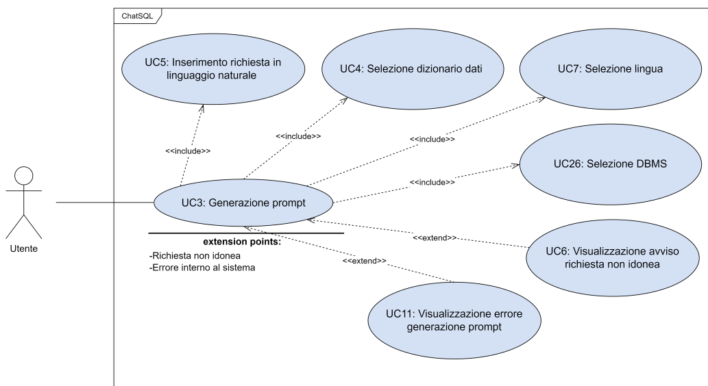
Figura 3.4: UC3
