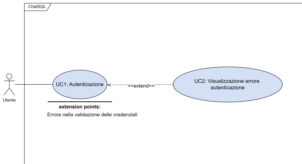
Figura 3.2: UC1
