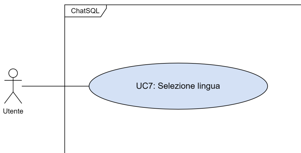
Figura 3.7: UC7
