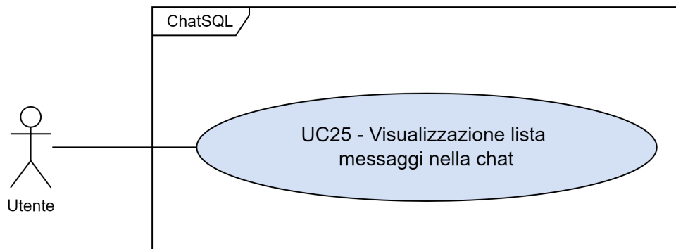
Figura 3.23: UC25
