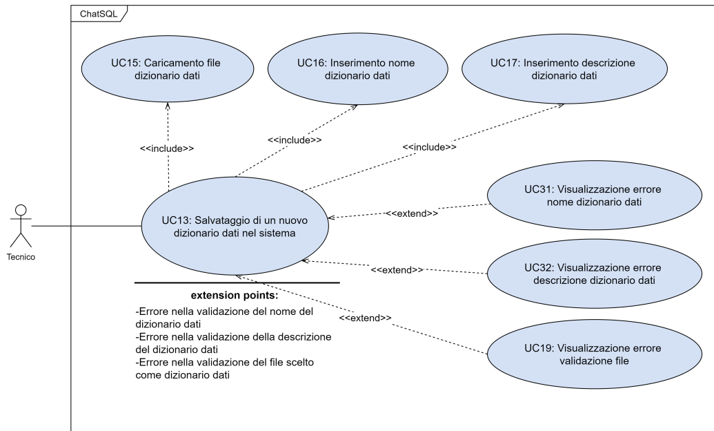
Figura 3.14: UC13
