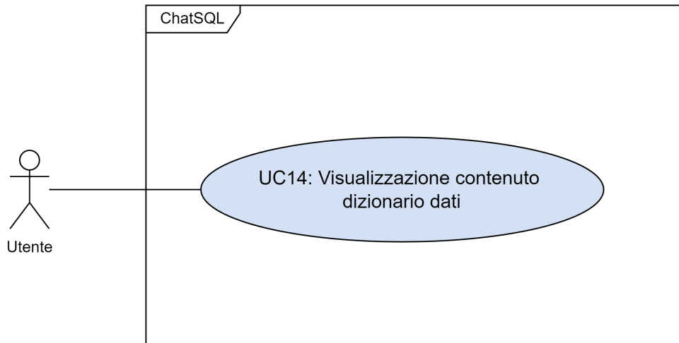
Figura 3.15: UC14
